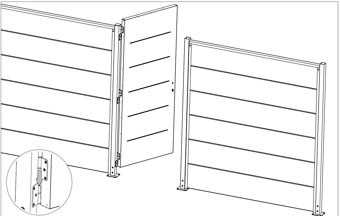
PORTE/POORT/DOOR/TOR
